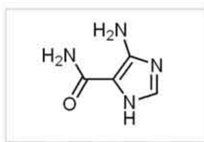
4-Aminoimidazole-5-carboxamide
