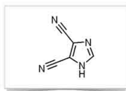
4,5-dicyanoimidazole
