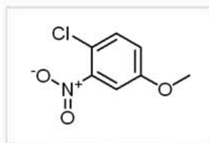
4-Chloro-3-Nitroanisole
