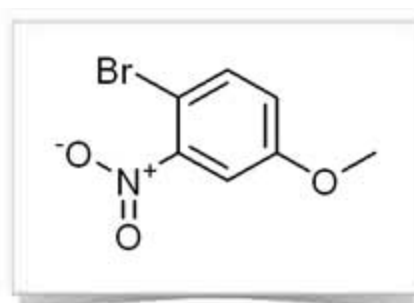
4-Bromo-3-Nitroanisole
